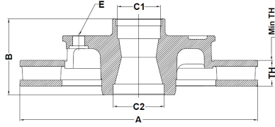
Disco de Freno
