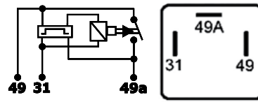
D0861 24V 3T
