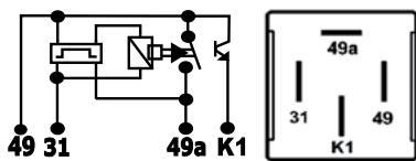
D0424S4 24V 4T C/S 500W
